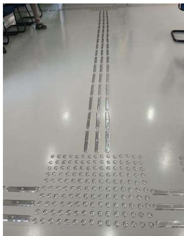
Foto 004 - Instalação de piso tátil “direcional”.
